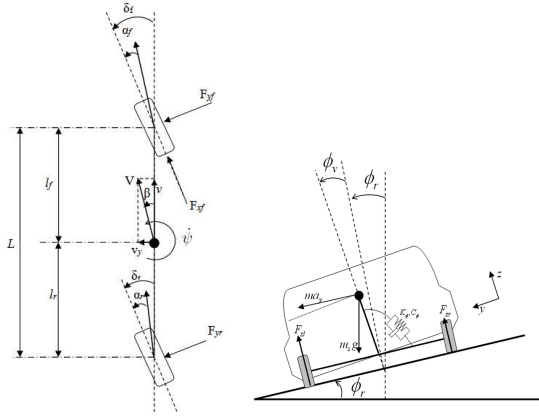
Figure 1 – Dynamique latérale et du roulis
