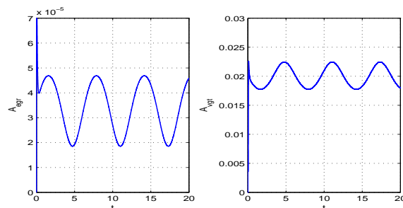
Figure 4 – Surfaces effectives des deux Vannes EGR et VGT
